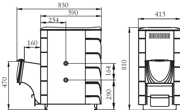
Рисунок 2. Габаритные размеры печи «Тунгуска 2011»
