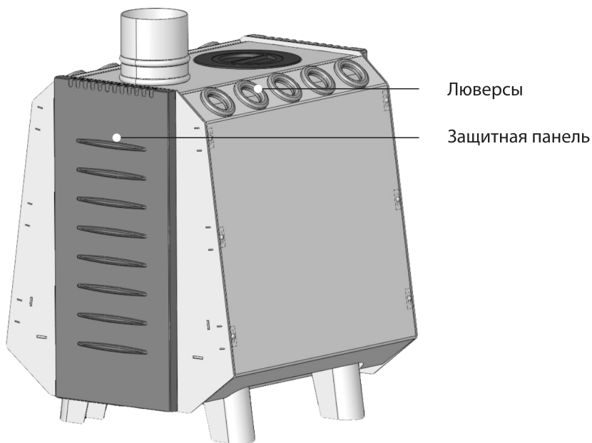
Рисунок 2. Конструкция печи Комбат (вид сзади)
